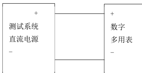
图 2 测试系统直流电压校准连接图
