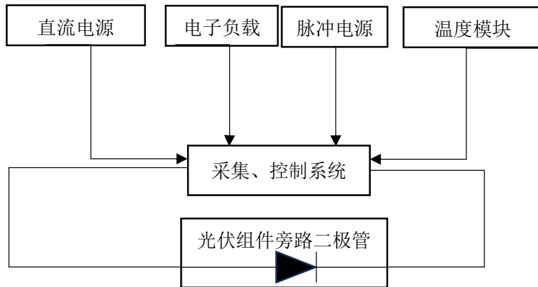
图 1 光伏组件旁路二极管测试系统原理图
